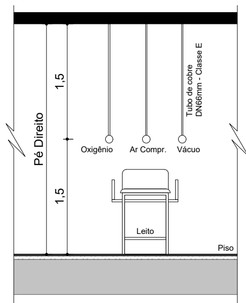
Vista Esquemática dos Pontos (Oxigênio, Ar Cond. e a Vácuo) Escala: 1:50
