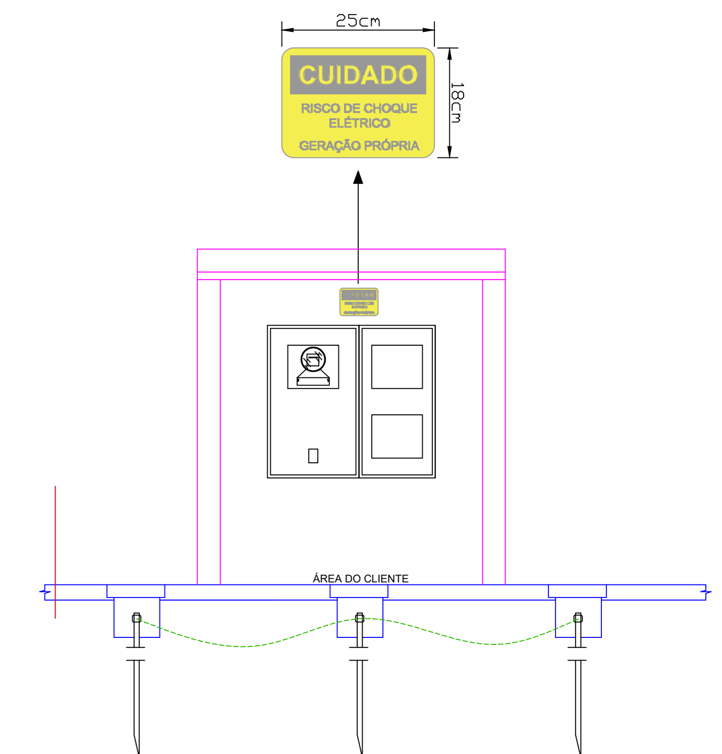
02 Detalhe Padrão de Entrada Placa de Advertência SEM ESCALA
